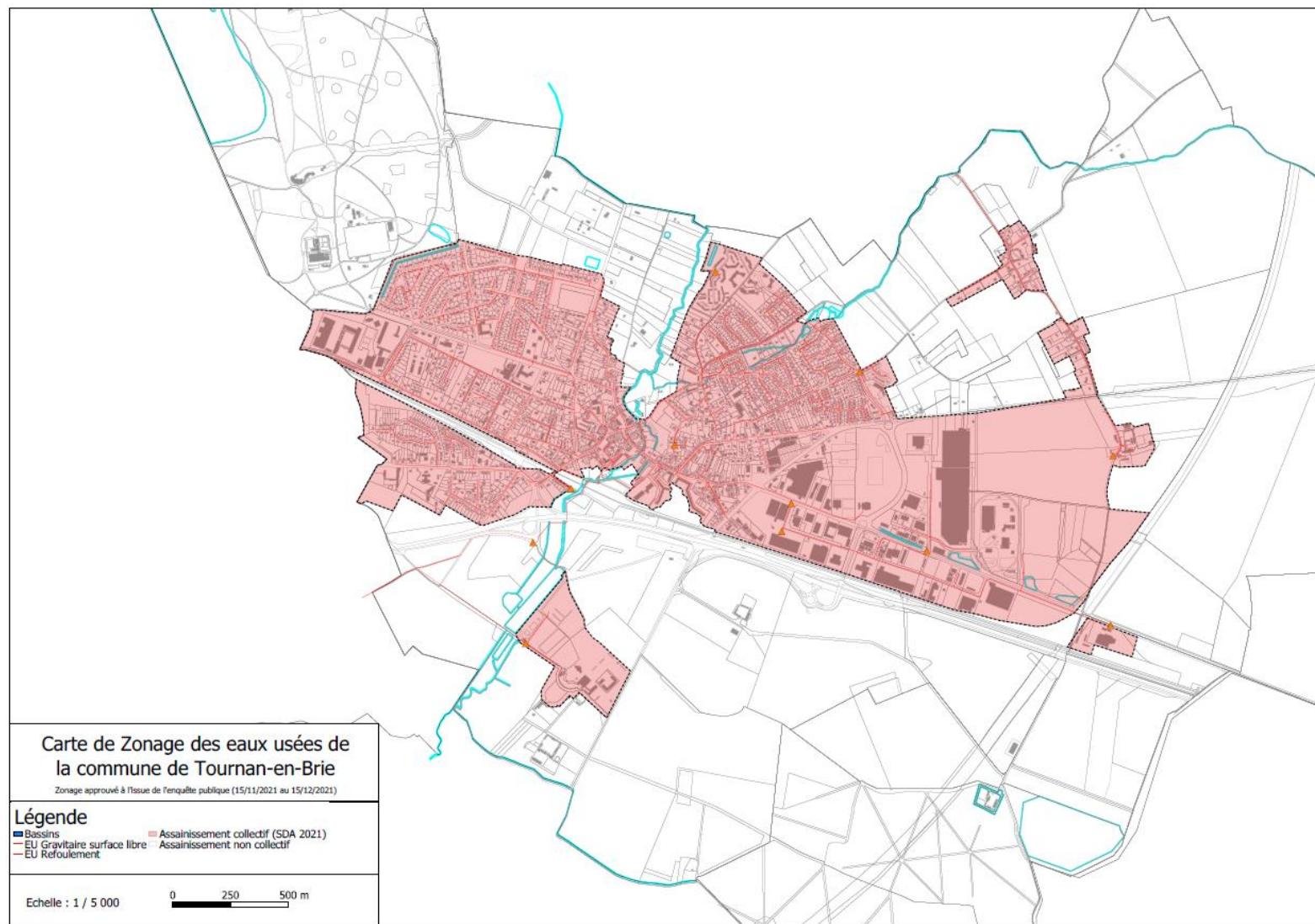
Figure 11 : Zonage des EU modifié - 2021
