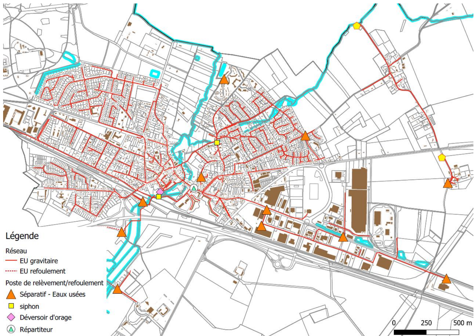
Figure 8 : Plan du réseau d'EU
