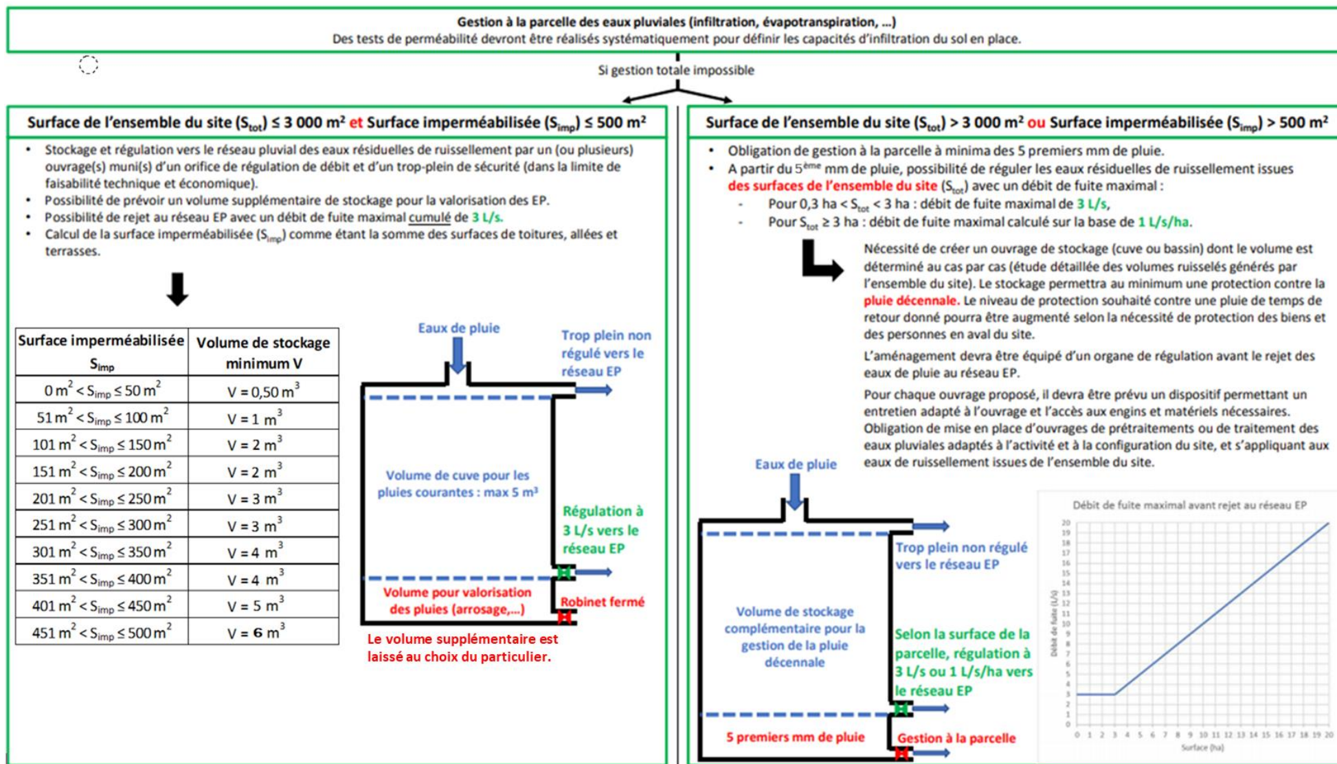
Figure 13 : Stockage et régulation des EP lorsque la gestion des EP à la parcelle n'est pas possible
