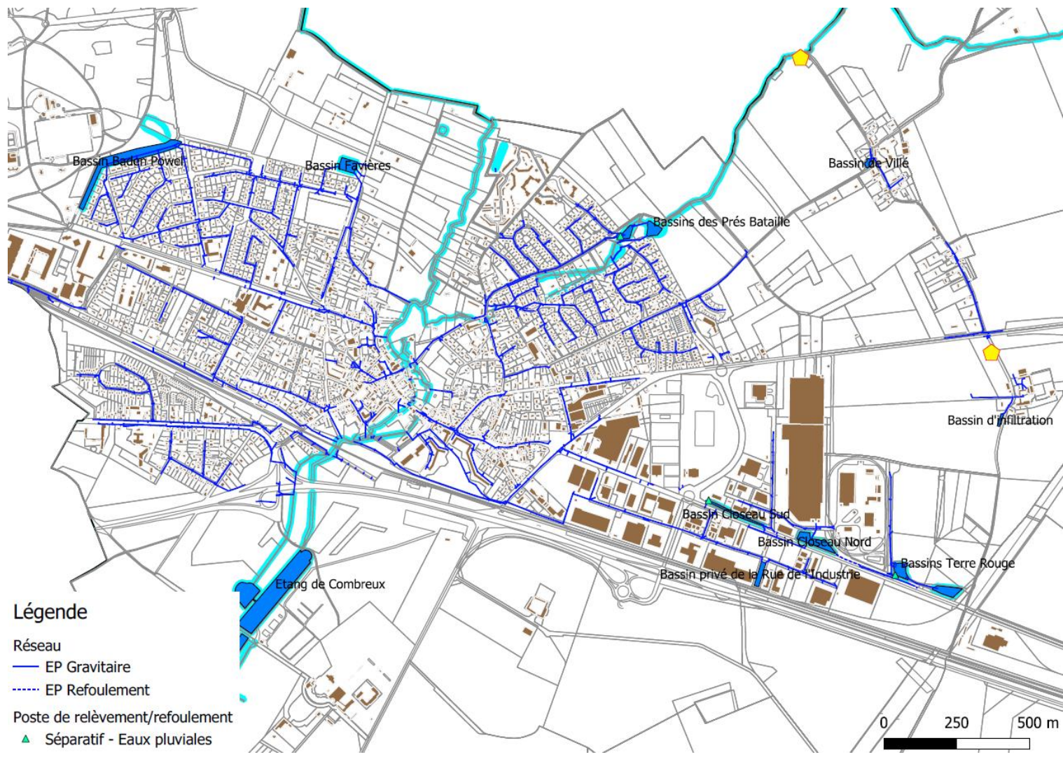
Figure 9 : Plan du réseau d'EP
